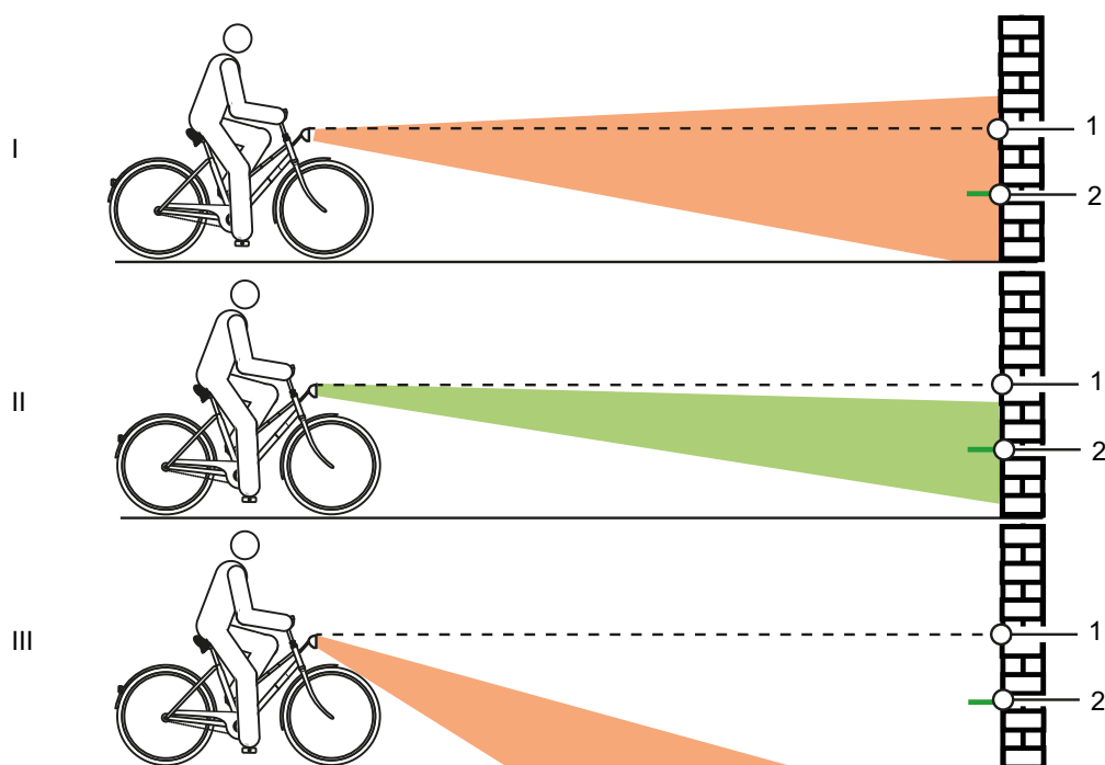
Figura 126: Luce regolata a un'altezza eccessiva (1), correttamente (2) e a un'altezza insufficiente (3)
