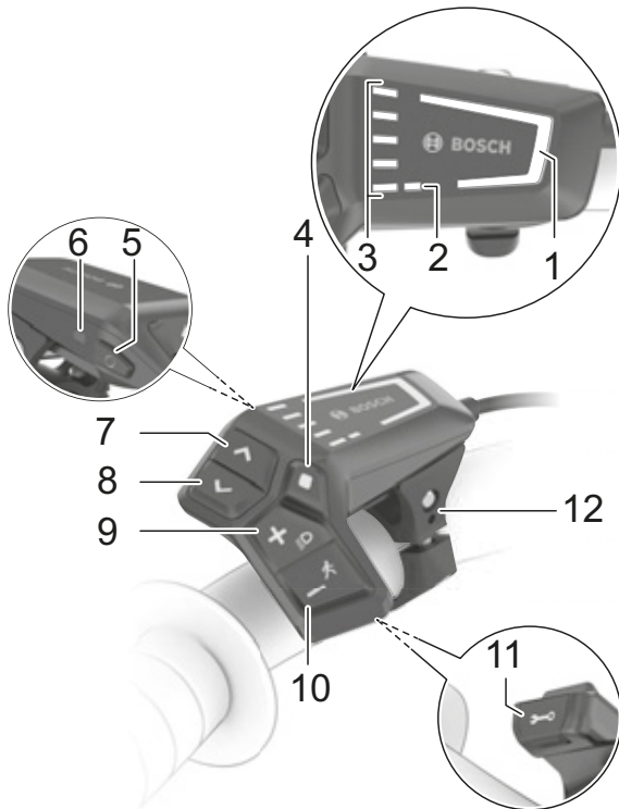
Figura 137: Schema del terminale di comando BOSCH LED Remote
