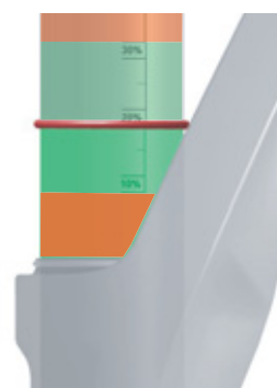
Figura 110: Intervallo prescritto della SAG (verde) e intervallo vietato della SAG (rosso)
