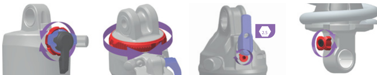
Figura 118: Ubicazione e forma del regolatore del rebound (rosso) in funzione del modello
