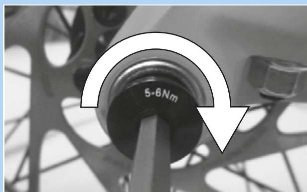
Figura 56: Serraggio della vite di sicurezza
