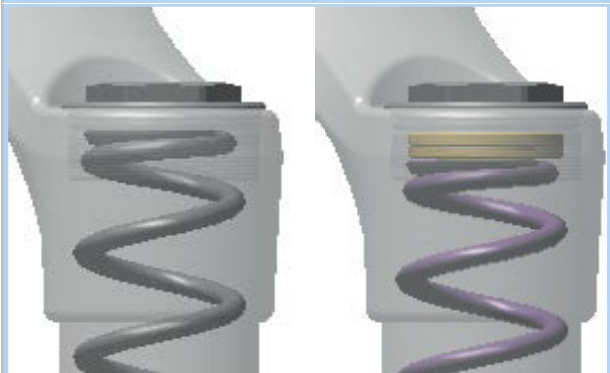
Figura 111: Avvitamento e svitamento dell'anello di regolazione del precarico
