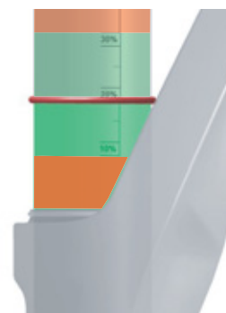
Figura 107: Intervallo prescritto della SAG (verde) e intervallo vietato della SAG (rosso)
