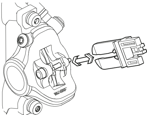
Figura 47: Fissaggio della sicura di trasporto
