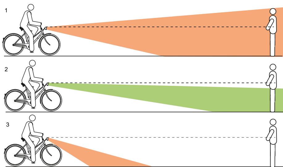
Figura 124: Luce regolata a un'altezza eccessiva (1), correttamente (2) e a un'altezza insufficiente (3)
