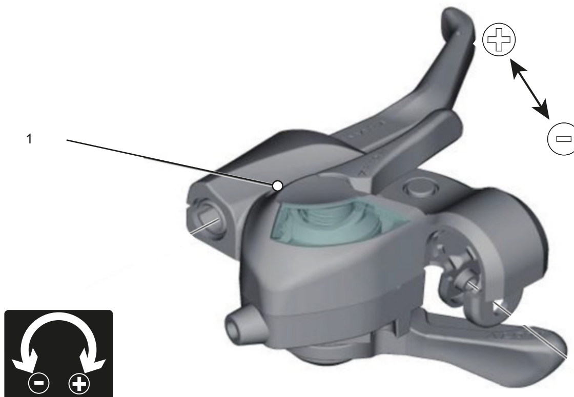
Figura 96: Posizione della vite di regolazione (1)
