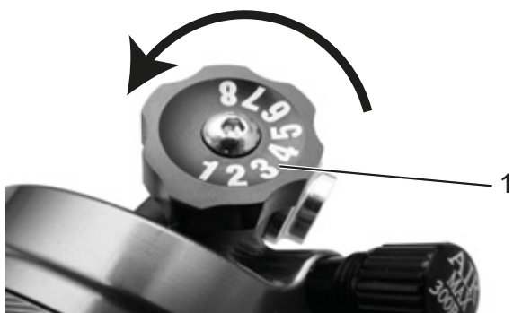
Figura 120: Regolatore dello stadio di compressione Suntour (1) sull'ammortizzatore del carro posteriore
