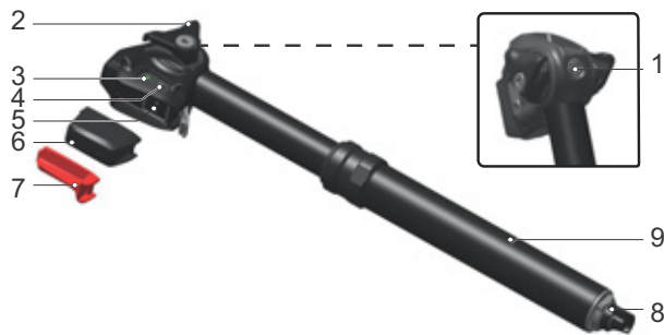
Figura 32: Struttura del cannotto reggisella ammortizzato ROCKSHOX Reverb AXS
