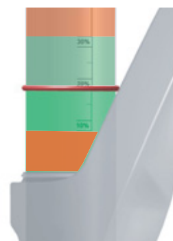
Figura 101: Intervallo prescritto della SAG (verde) e intervallo vietato della SAG (rosso)
