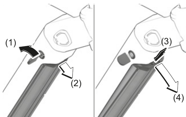
Figura 134: Smontaggio della batteria integrata
